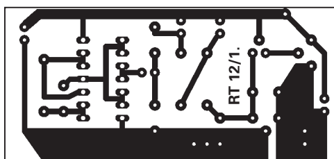
Stabilizált tápegység
