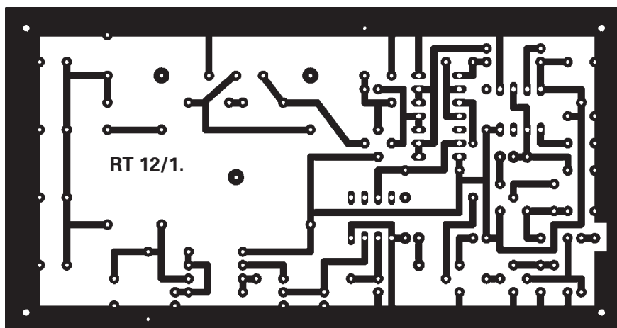
DC-DC konverter
