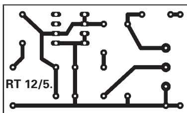
Varikapmérő előtét
