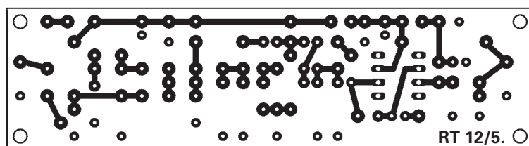
Mikrofonerősítő
