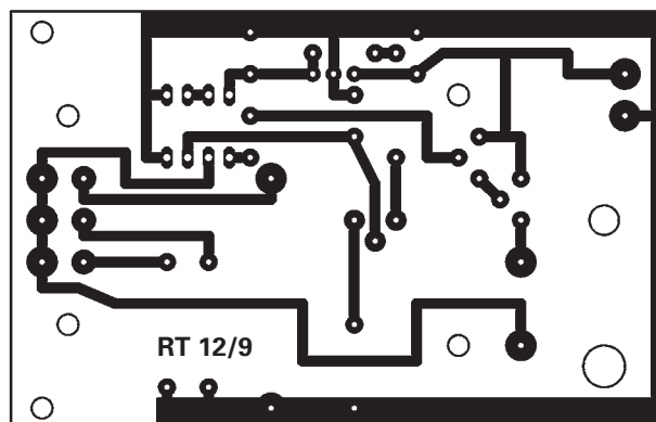
Milliohmmérő adapter
