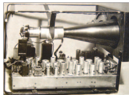
3. ábra. A már működő második tv-vevőm 1956-ból. 5BP4 sztatikus eltérítésű katód-sugárcsővel szuper rendszer, nem-intercarrier hangcsatornával
