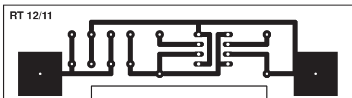
Tranzisztormérő előtét
