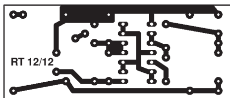
FET-es teljesítményszabályzó
