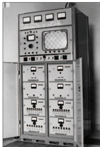
20. ábra. A BHG beadó mikró beltéri egységei. A dupla beépítés a „melegtartalék” képzése miatt volt szükséges
